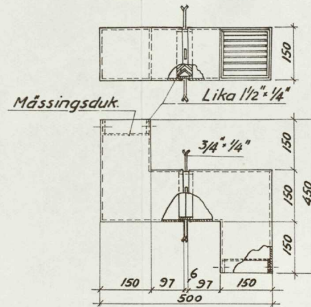
Ammunitionsmagasin i betongkonstruktion. Mätt i millimeter.
