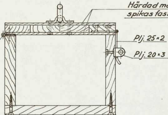
Sektion A-A.
