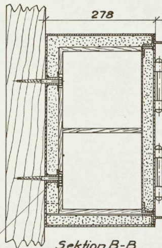
Sektion B-B
