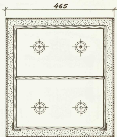
Sektion A-A
