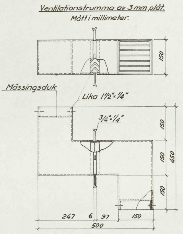
Sprängämnesmagasin i betongkonstruktion. Mått i millimeter.
