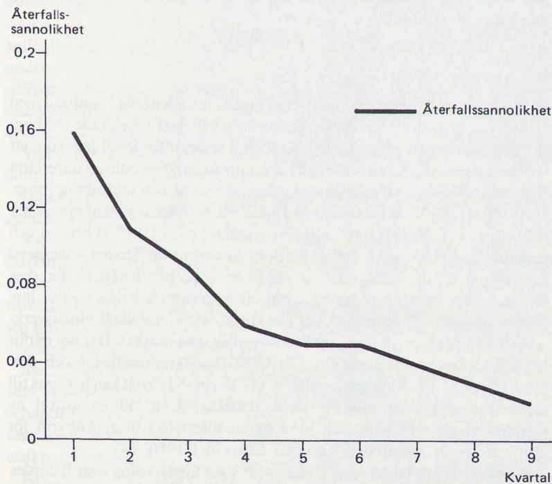
Diagram 1. Återfallssannolikhet vid olika tidpunkter.
